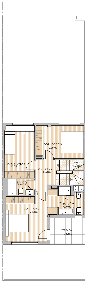
PLANTA PRIMERA
